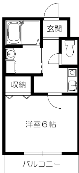
01号室 (22.68㎡)
