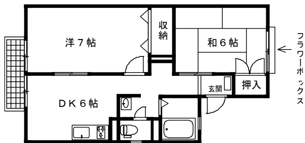
A Type (専有床面積/45.31㎡)
